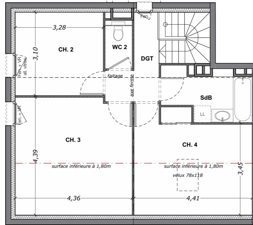
PLAN DU NIVEAU 2
