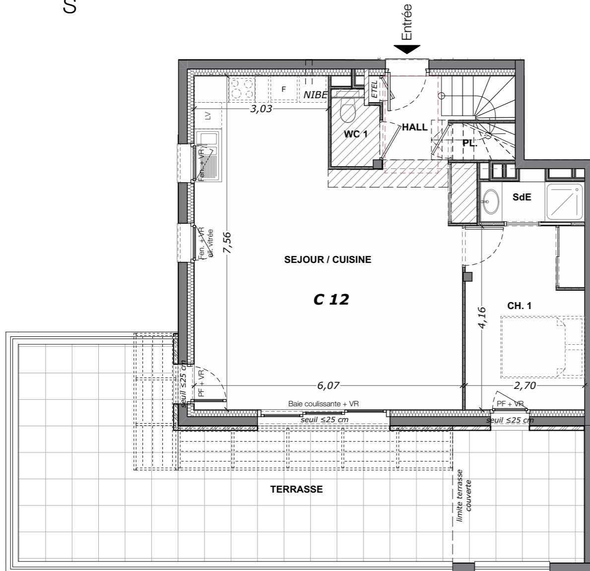
PLAN DU NIVEAU 1
